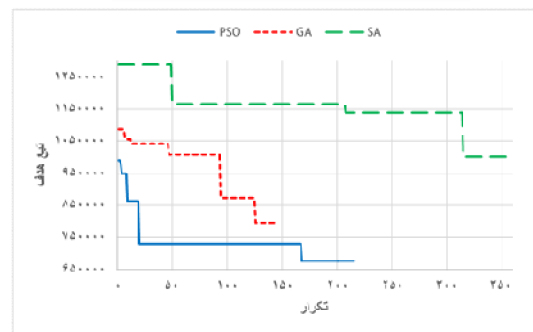
زیرمساله ۴
