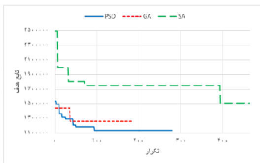
زیرمساله ۳
