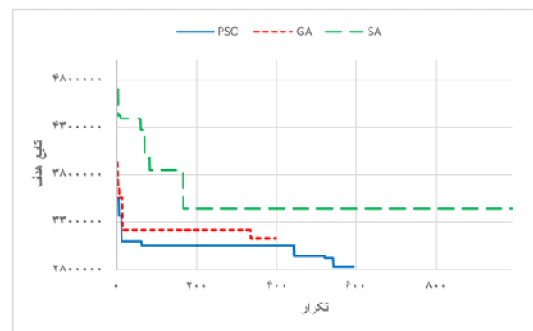
زیرمساله ۸
