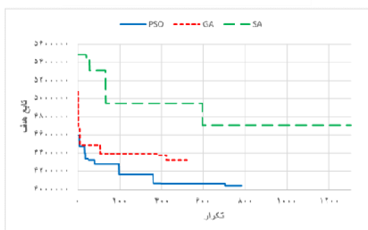
زیرمساله ۷
