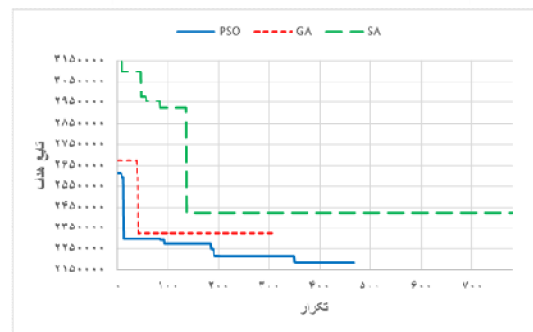
زیرمساله ۶
