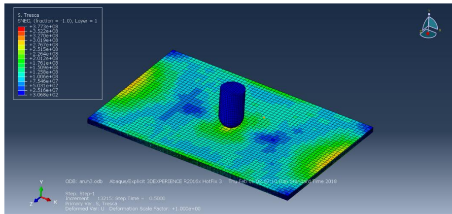
شکل ۱۳. مدل المان محدود ترکیب جدید گالر تحت ضربه
