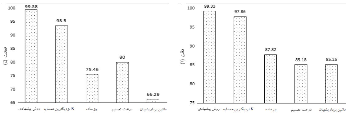
شکل ۴. مقایسه میزان دقت و صحت روش پیشنهادی با سایر روش‌ها
