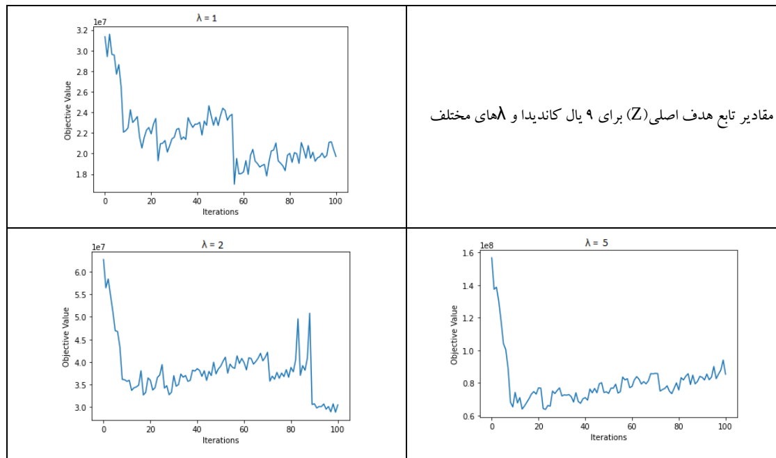
شکل ۷. مقادیر تابع هدف اصلی (Z) برای ۹ یال کاندیدا و \lambda های مختلف در شبکه سیوکس فالز
