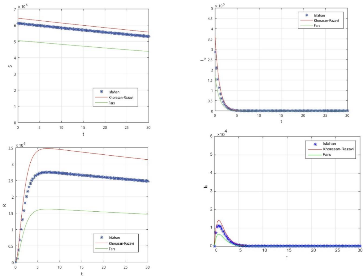
شکل ۴. نمودارهای S ، I_k و R در سه استان با کنترل با استفاده از داده‌های جدول ۲
