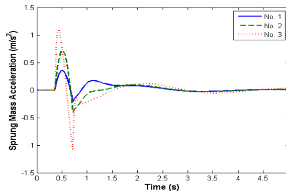
شکل ۱۱. نمودار شتاب جرم فربندی شده بر حسب زمان؛ بهینه شده توسط روش ازدحام ذرات در ۳ نقطه طراحی مختلف
