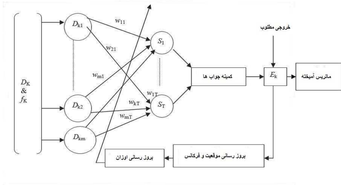
شکل ۴. الگوریتم بت
