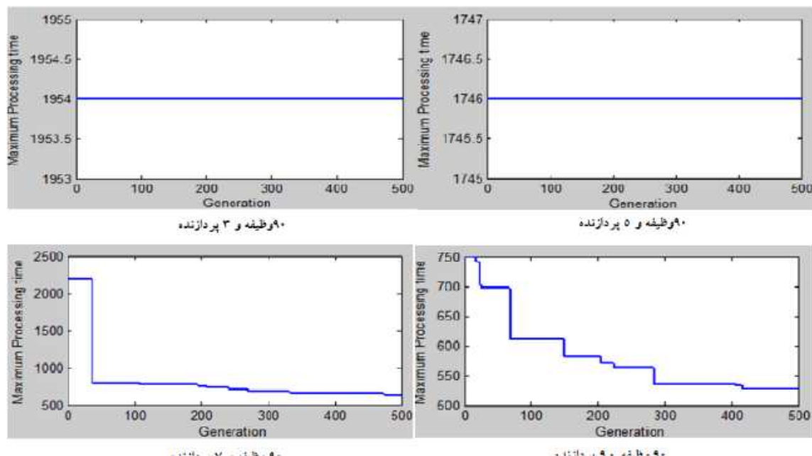
شکل ۱۶. نمودار زمان اجرای گراف ۹۰ وظیفه‌ای با تعداد پردازنده‌های مختلف با الگوریتم لیست
