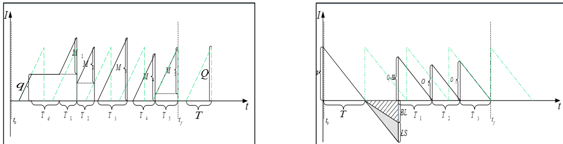
شکل ۳. نمودار وضعیت گردش موجودی در تولیدکننده (سمت چپ محصول و سمت راست مواد اولیه)
