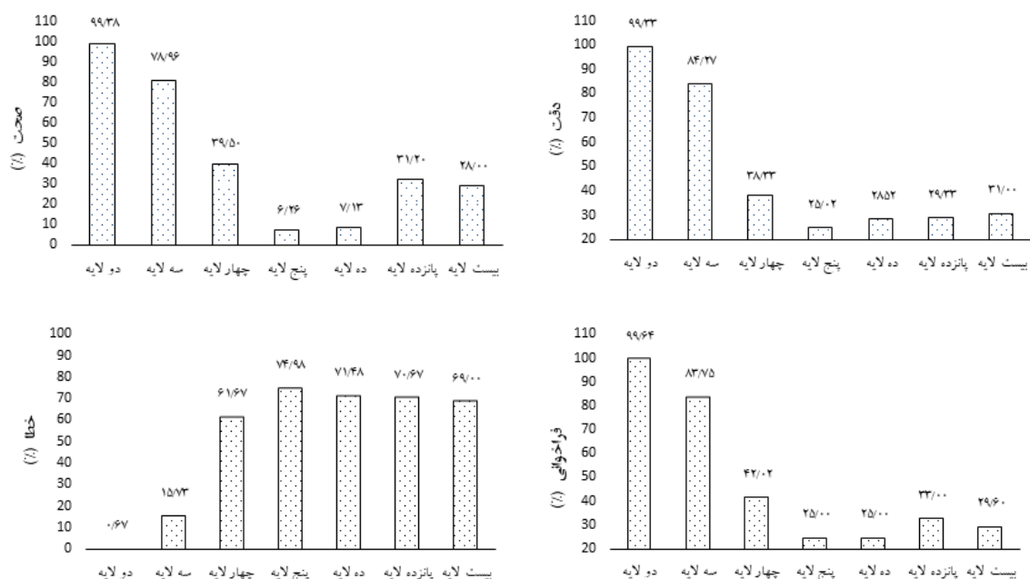
شکل ۳. مقایسه میزان دقت، فراخوانی، صحت و خطای شبکه عصبی با تعداد لایه‌های مختلف
