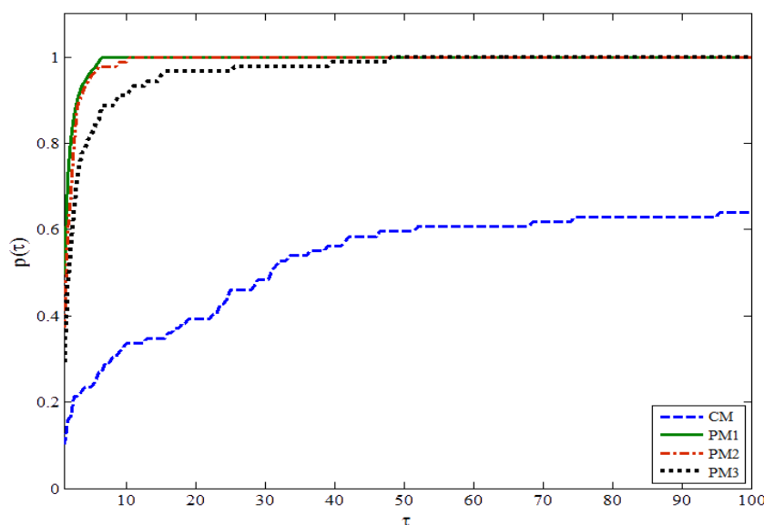
شکل ۱. نمودارهای عملکرد الگوریتم‌های CM، PM1، PM2، PM3 و PM3 با معیار خطای میانگین
