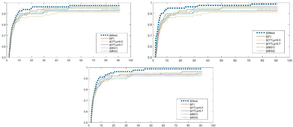
شکل ۳. نمودار عملکرد زمان پردازنده (بالا سمت راست: \rho_k = 0.7 و u_k = S_k ، بالا سمت چپ: \rho_k = 0.8 و u_k = S_k ، پایین: \rho_k = 0.8 و u_k = y_k )
