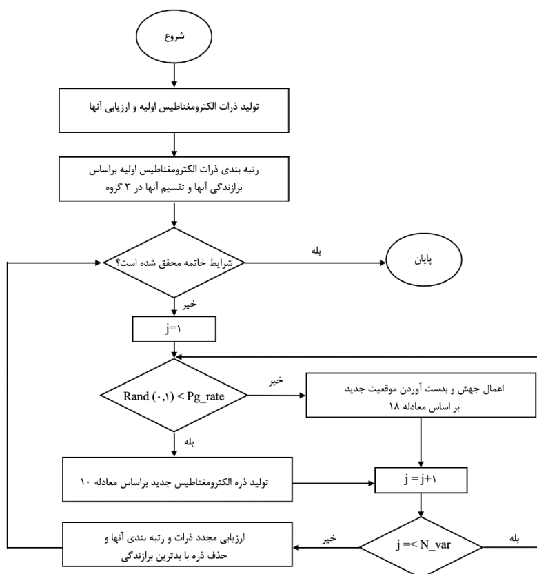
شکل ۳. روندنمای الگوریتم پیشنهادی
