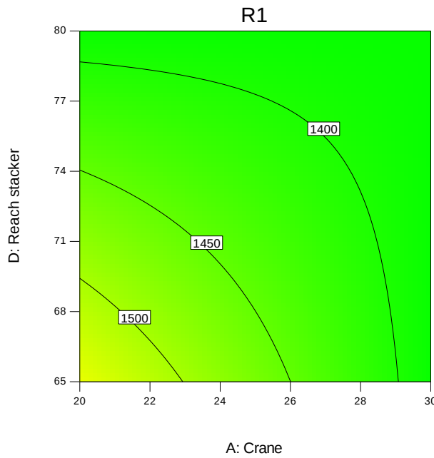
شکل ۷. مقایسه فاکتور جرثقیل با ریچ استکر
