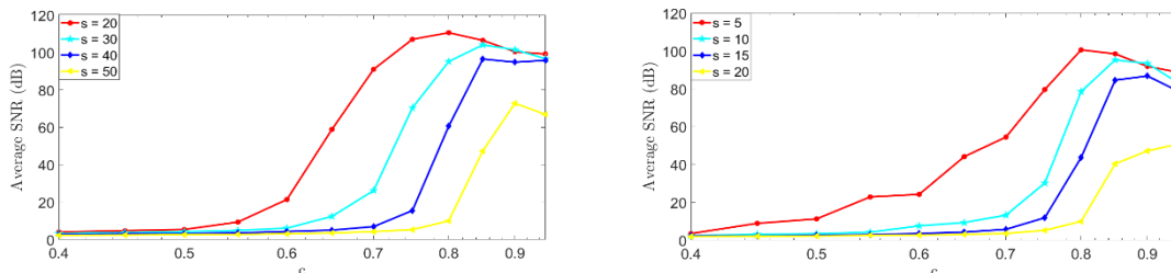
شکل ۲. میانگین شاخص SNR روش پیشنهادی برای ماتریس در ابعاد A_{50 \times 150} (سمت راست) و A_{200 \times 100} (سمت چپ)
