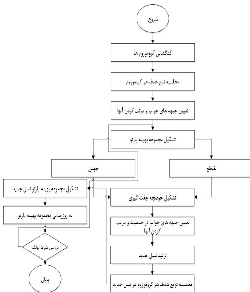
شکل ۲. فلوچارت اجرایی الگوریتم NSGA-II
