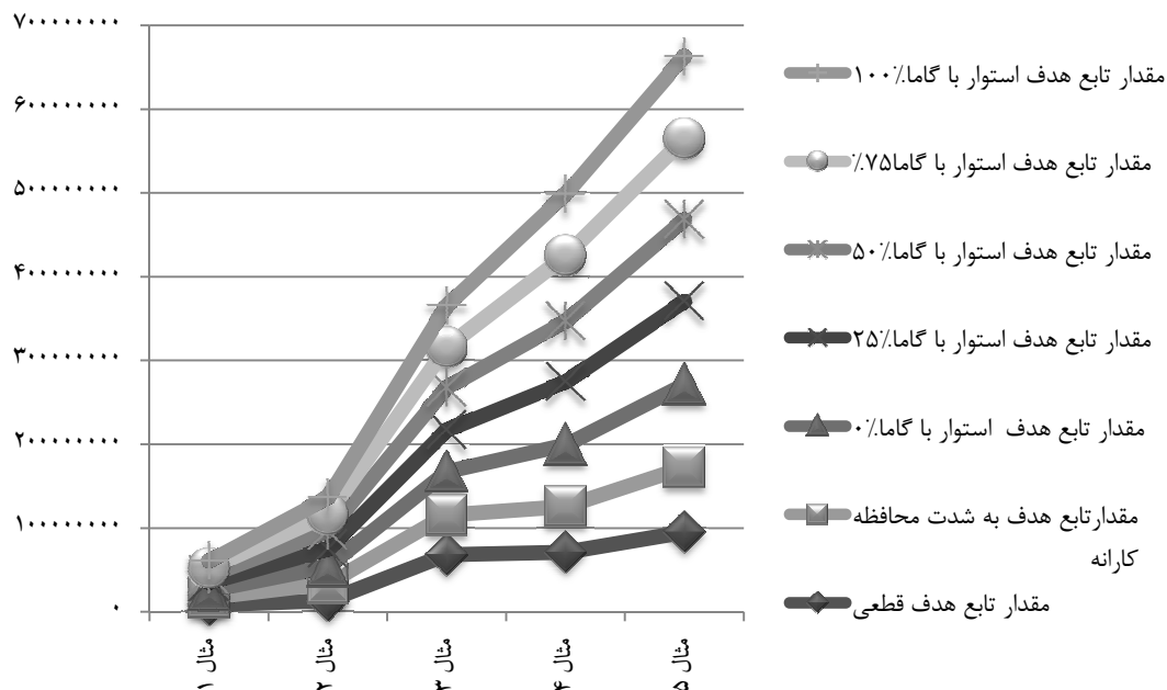
شکل ۱. مقایسه مقادیر تابع هدف قطعی با دو رویکرد استوار (اولین مثال با اولین بعد جدول (۴) مطابقت دارد)
