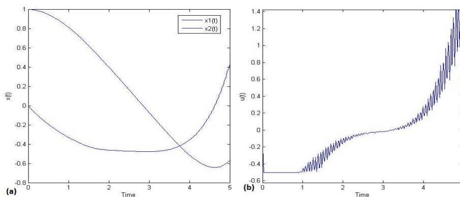
شکل ۲. نمودار جواب‌های بهینه‌ی مساله‌ی ۶-۲: (a) منحنی‌های حالت بهینه (b) منحنی کنترل بهینه
